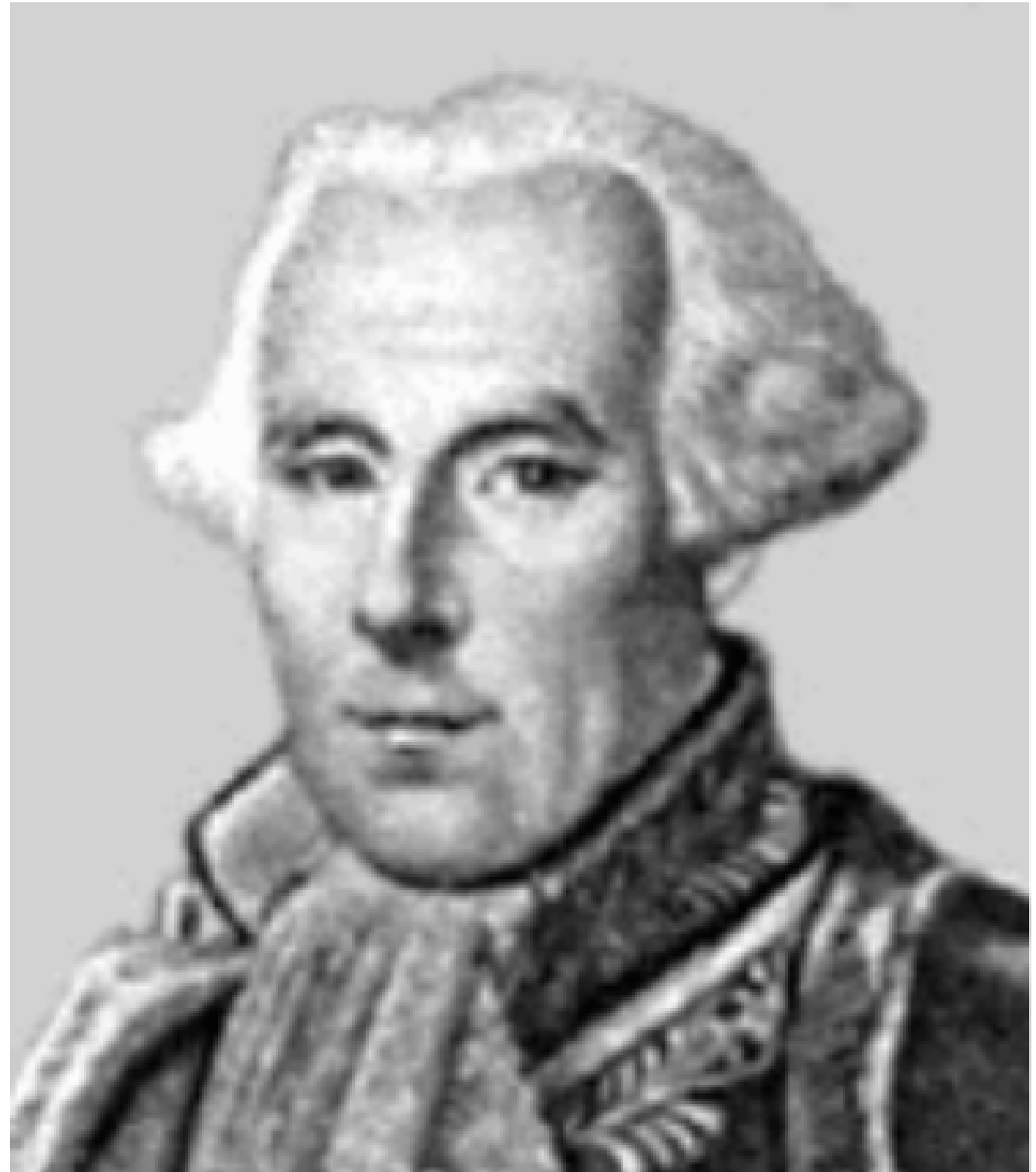
Felix Savart 1791-1841
