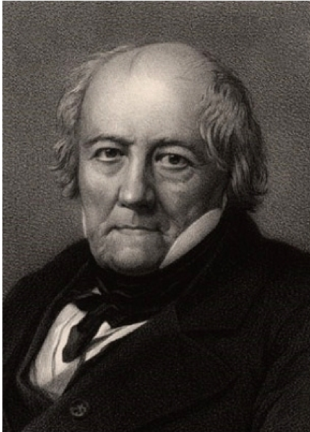
Jean-Baptiste Biot 1774-1862
