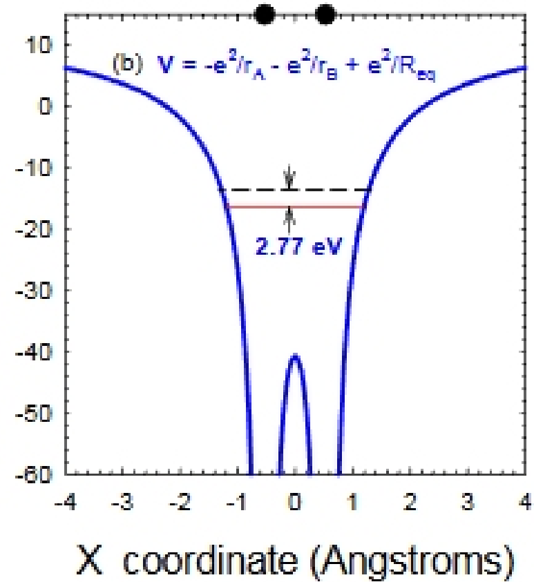
H 2 + molecule
