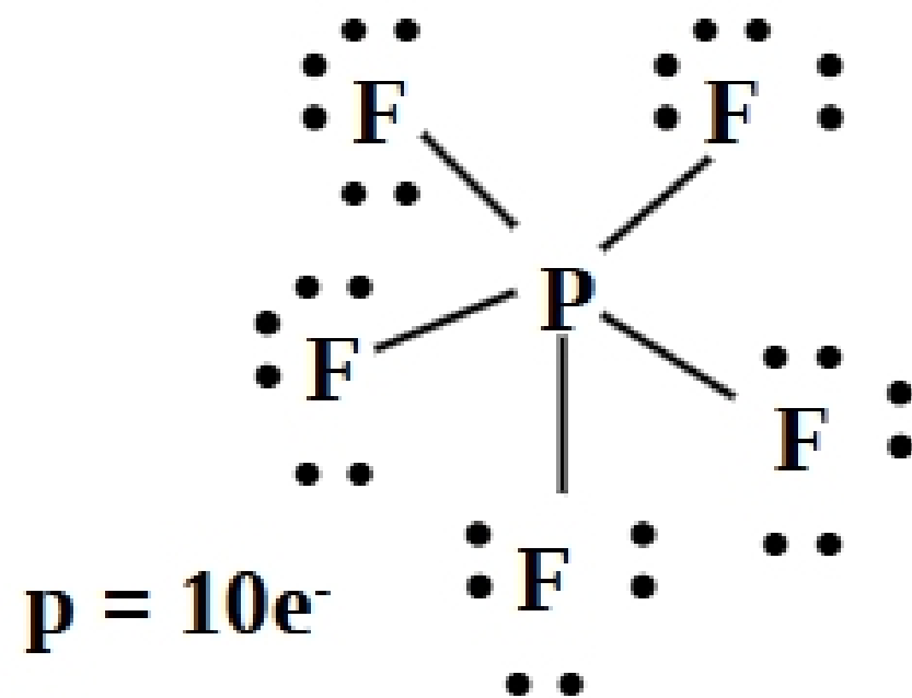
Phosphorous pentaffluoride
